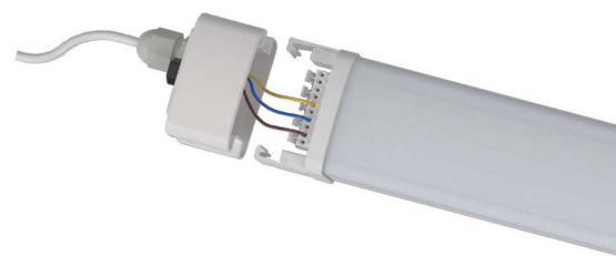
Detachable Endcap
